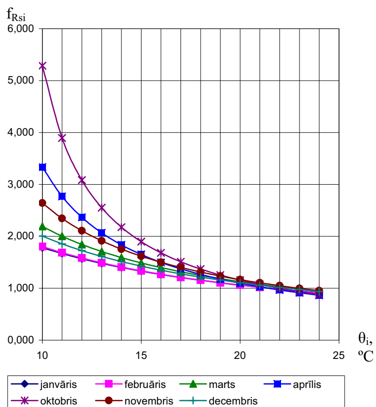
4-4.att. Korozijas riska novērtējums 4.klases telpās
