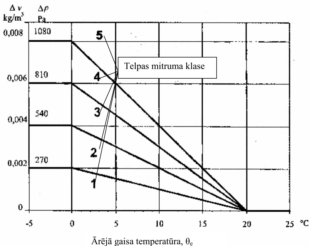
3-1.att. Ārējā un iekšējā gaisa ūdens tvaika parciāla spiediena starpība \Delta p , Pa un gaisa mitruma satura starpība \Delta v , kg/m³ atkarībā no ārējā gaisa temperatūras
