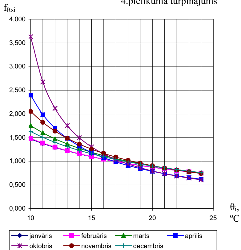
4-3. att. Sēnīšu augšanas riska novērtējums 4.klases telpās
