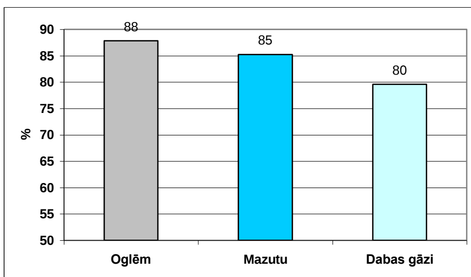
Attēls 1.2.3.: Emisiju procentuālais ietaupījums izmantojot enerģētisko koksni (šķelda, mitrums W=35\% , KI=0,82 ) salīdzinājumā ar fosilajiem energoresursiem.
