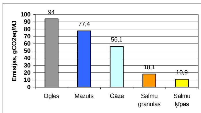
1.2.7.attēls. Salmu ķīpu, salmu granulu un fosilo kurināmo izmantošanas emisijas siltuma enerģijas ražošanai.
