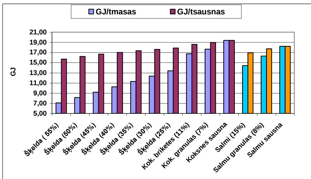
1.2.5.attēls. Dažāda mitrumu koksnes un salmu kurināmo 1 tonnas masas un 1 t nosacītās sausnas (1 t sausnas un mitrums) sadedzināšanas enerģijas.
