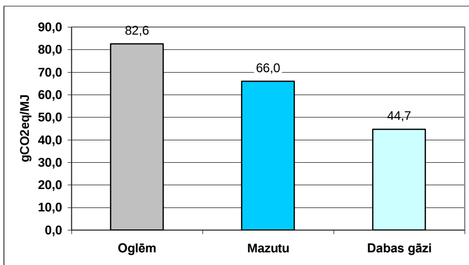
Attēls 1.2.2. Emisiju ietaupījums izmantojot enerģētisko koksni salīdzinājumā ar fosilajiem energoresursiem.
