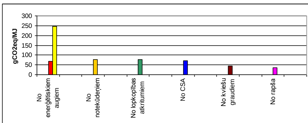
1.6.4. attēls. Rangs atkarībā no SEG emisiju ietaupījuma pret mazutu.
