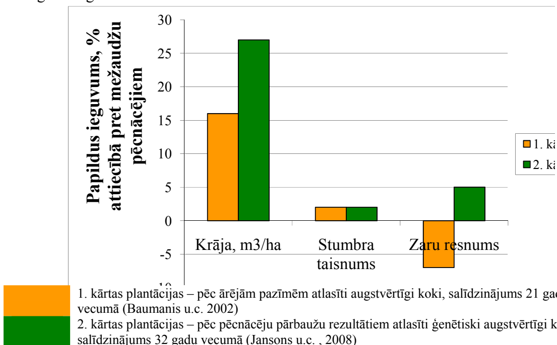
1.2. attēls. Priedes sēklu plantāciju pēcnācēju pārākums pār mežaudžu pēcnācējiem Latvijas rietumu daļā.
